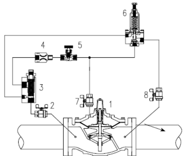
Schematic A-0423F
